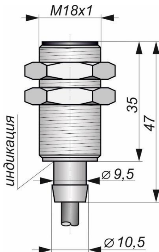
Габаритный чертеж
